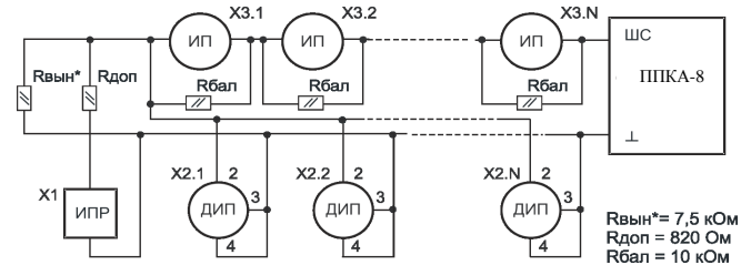
Рис.5. Комбинированная схема включения ШС со сработкой по одному извещателю (с перезапросом).
