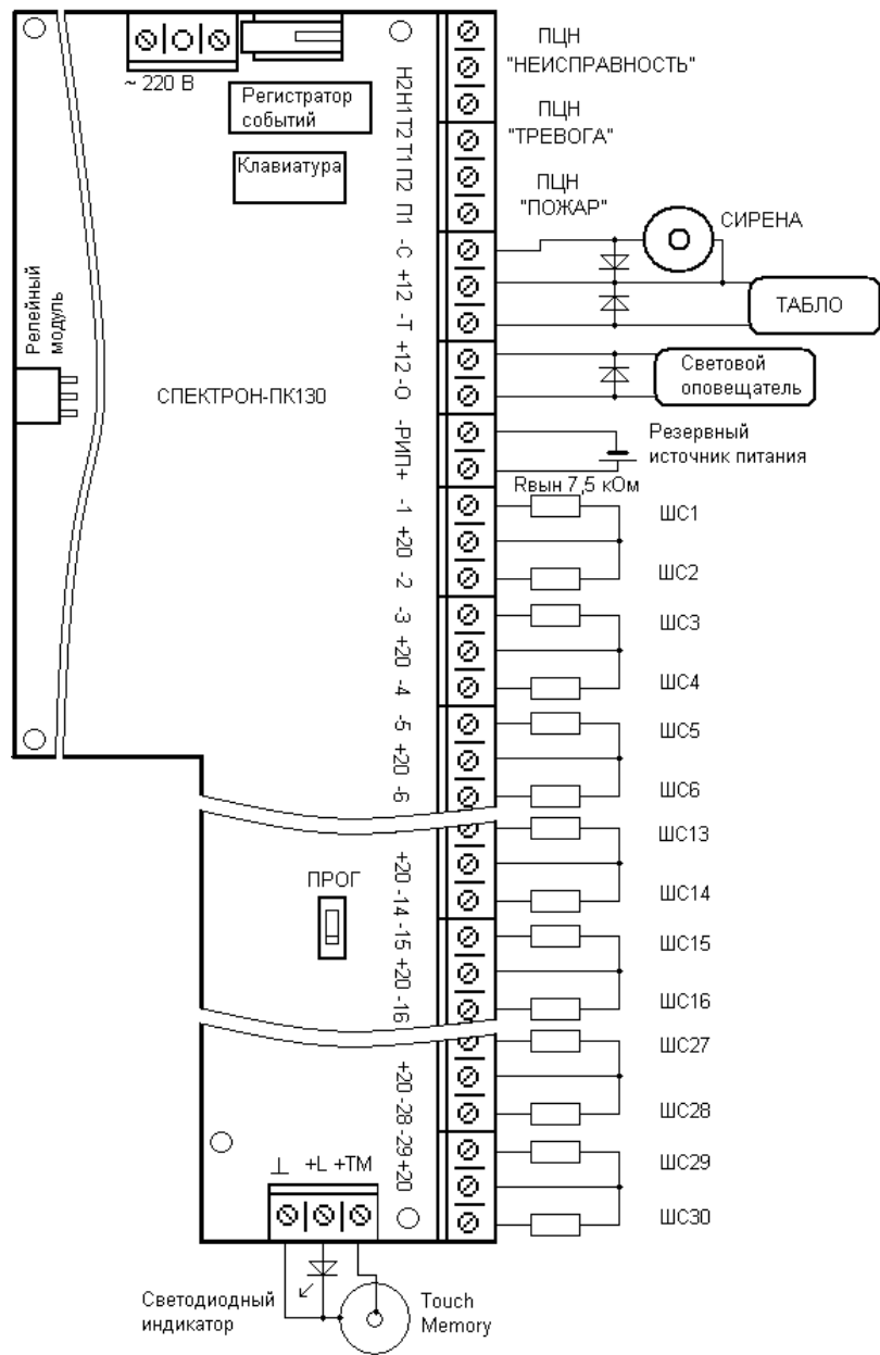
Рис.2. Схема внешних соединений прибора ППКА-30.
