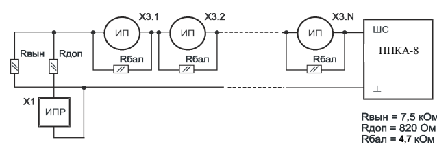
Рис.4. Схемы включения ШС с несколькими тепловыми извещателями (типа ИП-105) и сработкой по двум извещателям (с перезапросом).
