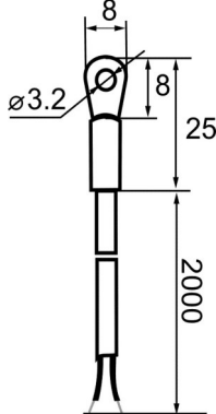
Габаритные размеры датчика (заказывается отдельно)
