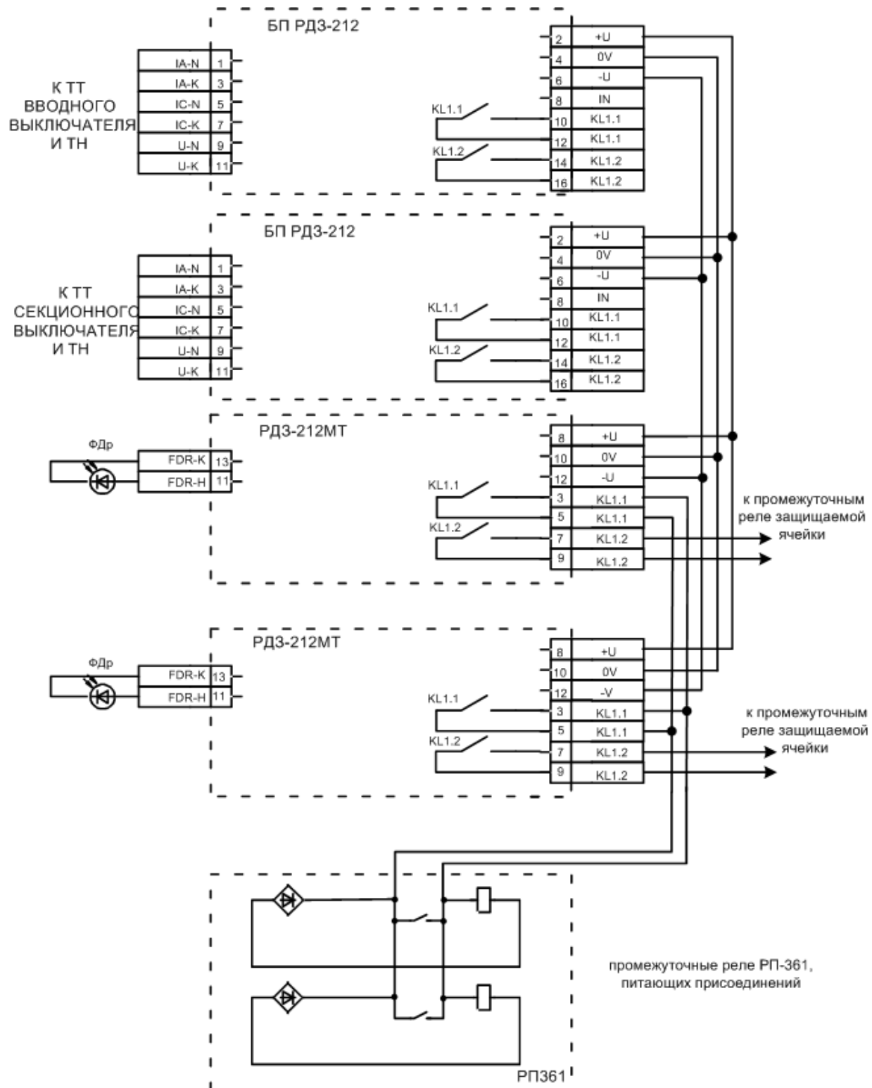
Рис.3. Схема подключения
