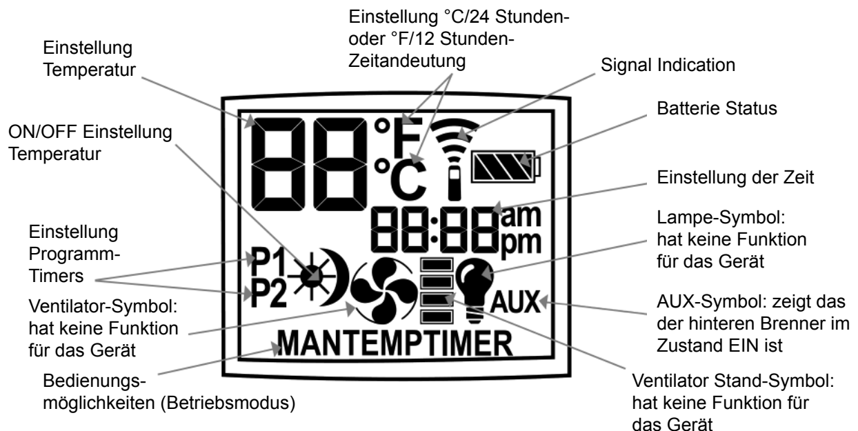
Abbildung 2: Display Handsender
