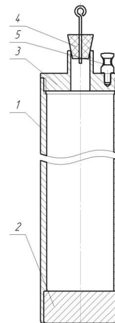
Рис. 1.2.3.Пробоотборник типа ППА. 1 – корпус; 2 – донце; 3 – крышка с воздушным штуцером для пробы; 4 – пробка со штоком для крепления металлического троса; 5 – бобышка для крепления троса.
