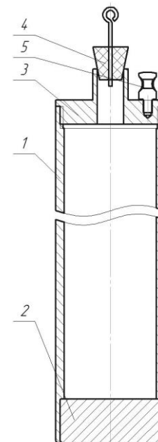
Рис. 1.2.3.Пробоотборник типа ППА. 1 – корпус; 2 – донце; 3 – крышка с воздушным штуцером для пробы; 4 – пробка со штоком для крепления металлического троса; 5 – бобышка для крепления троса.
