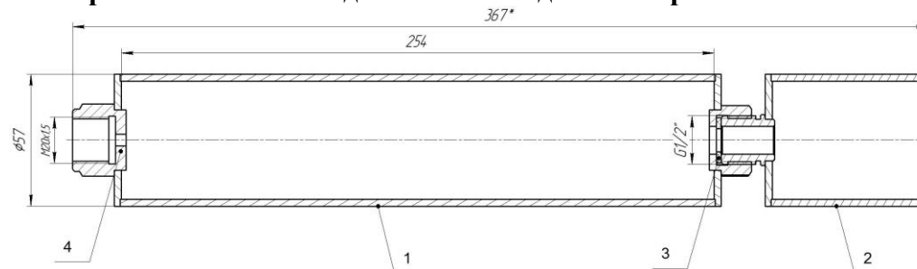
Рис. 1 Бомба Рейда БР-010М с одним отверстием: 1 – воздушная камера; 2 – жидкостная камера; 3 – уплотнение между воздушной и жидкостной камерой; 4 – штуцер для присоединения манометра.
