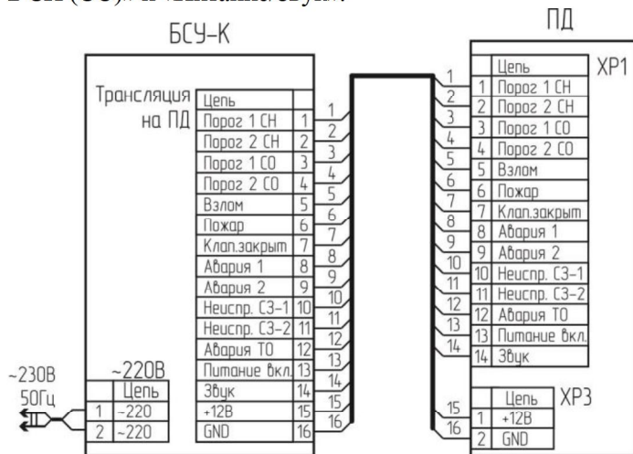
Рисунок 1 – Схема подключения
