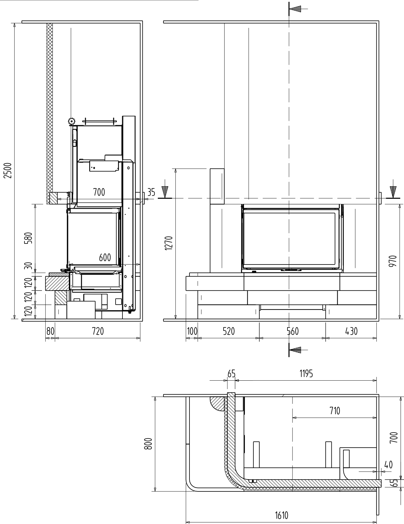
Plan d'implantation / Layout drawing / Einbauplan
