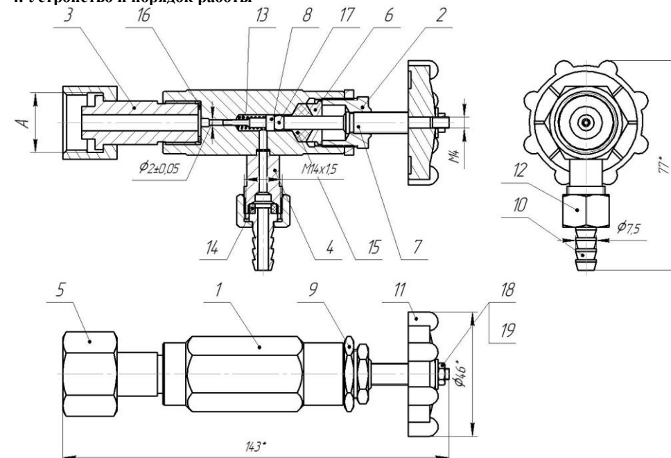
Рис. 1. Вентиль точной регулировки ВТР-1 1 – корпус; 2 – гайка; 3 – штуцер присоединительный; 4 – штуцер шланговой надставки; 5 – гайка накидная; 6 – буksа; 7 – штоk; 8 – золотник; 9 – гайка поджимная; 10 – шланговая надставка (ёрш); 11 – вороток; 12 – гайка надставки поджимная; 13 – пружина возвратная; 14 – уплотнение шланговой надставки; 15 – сальник; 16 – уплотнение штуцера; 17 – шарик штока; 18 – шайба; 19 – гайка.
