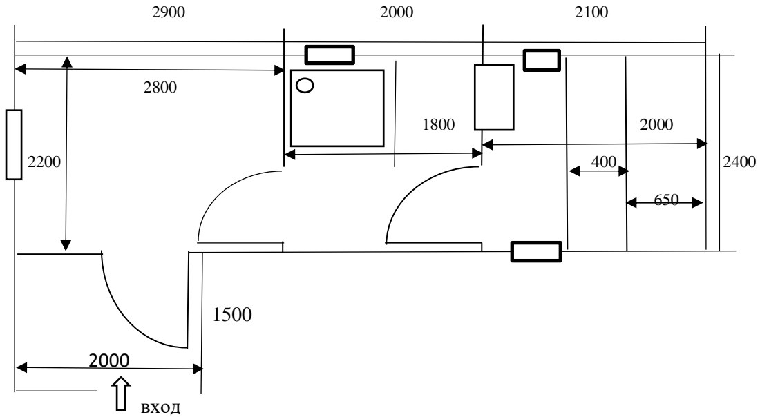
Арт. 244 Мобильная баня р-р 7000х2400 мм с крыльцом р-р 2000х1500 мм План-схема мобильной бани деревянной р-р 7000х2400 мм (возможно сделать баню в зеркальном изображении)
