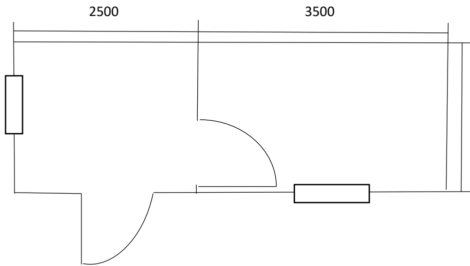
План-схема бытовки «Домик для лета» р-р 6000х2450 мм
