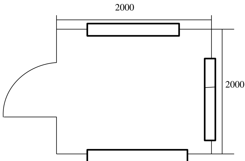
Спецификация на будку для охраны р-р 2000х2000 мм, арт. 135
