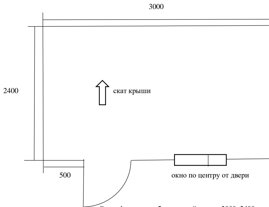
Спецификация на блок-контейнер р-р 3000x2400 мм, арт. 297
