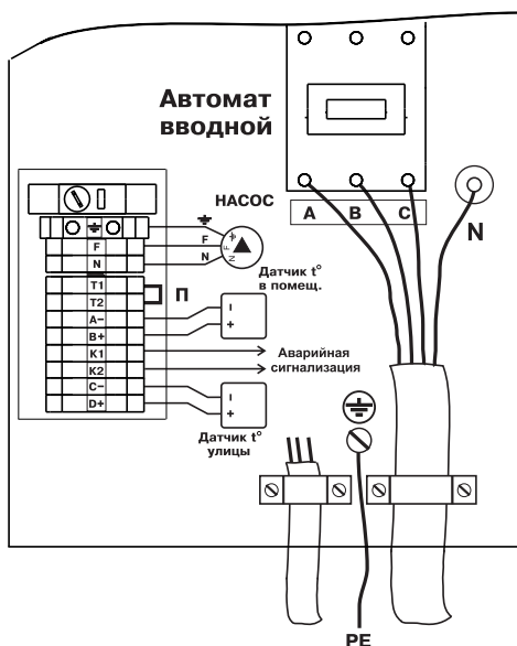
Рис. 3 Схема подключения электроводонагревателя
