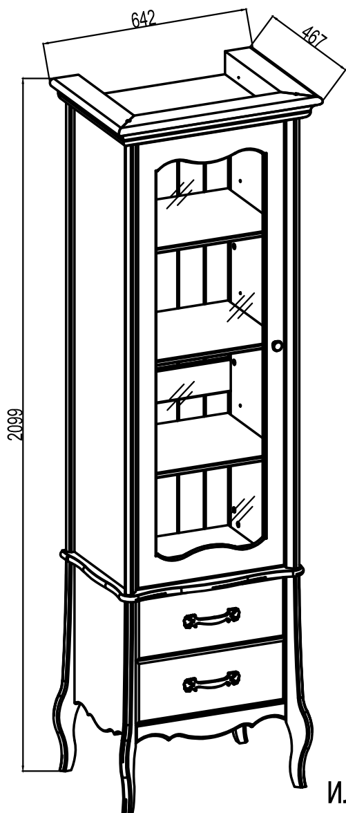
Исполнение А.
