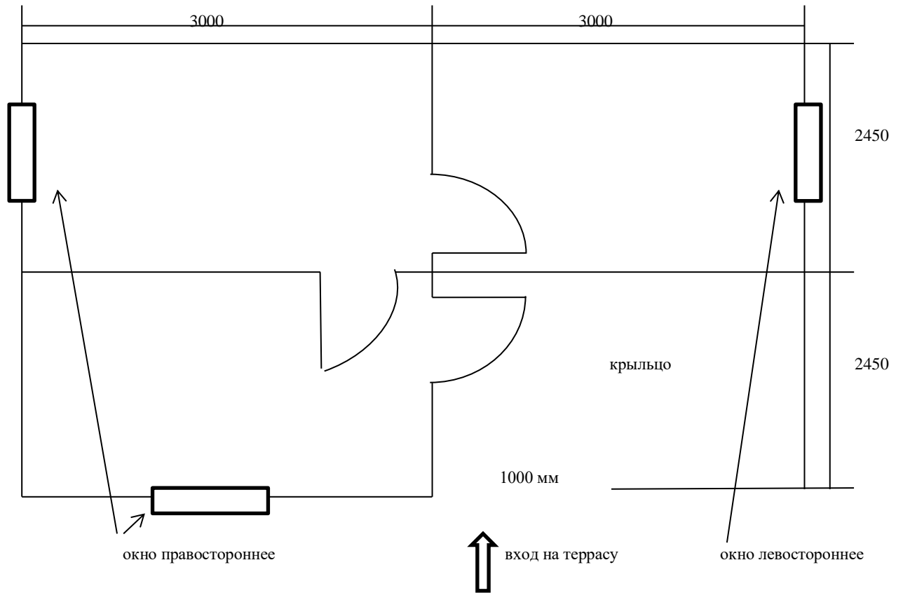
Арт.114 План-схема садового домика р-р 6000х4900 мм
