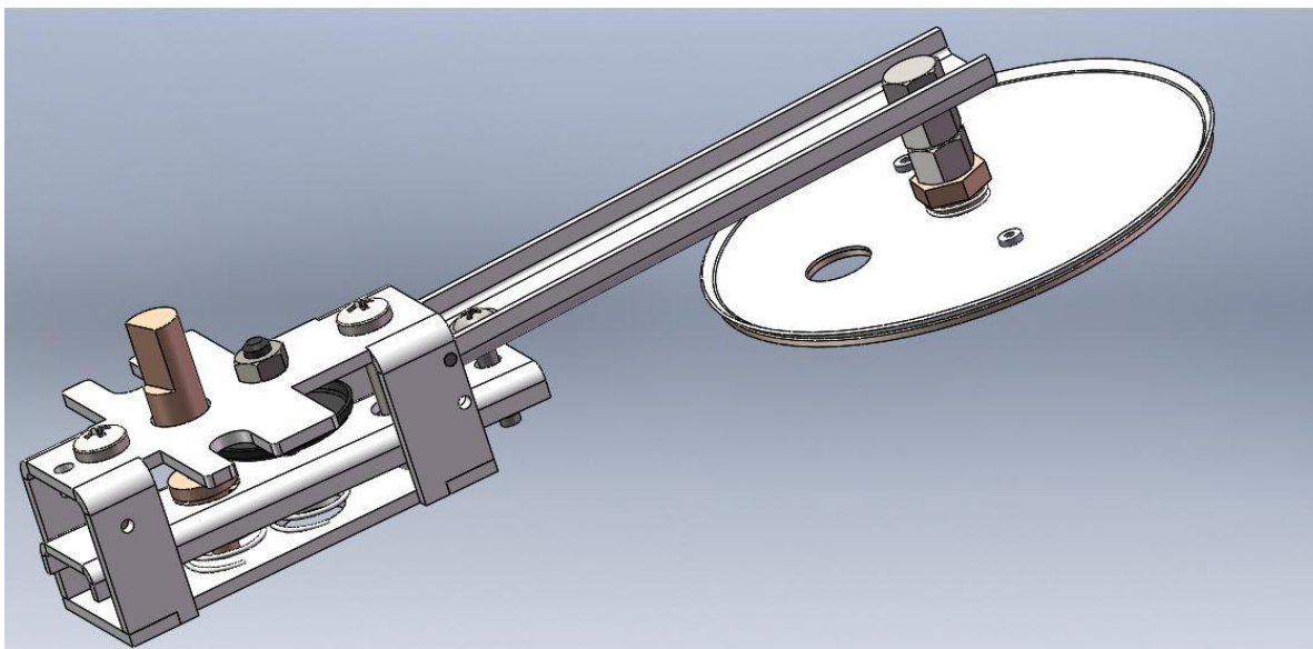
Автоматический механизм для первичного и вторичного воздуха (термостат твердого топлива)
