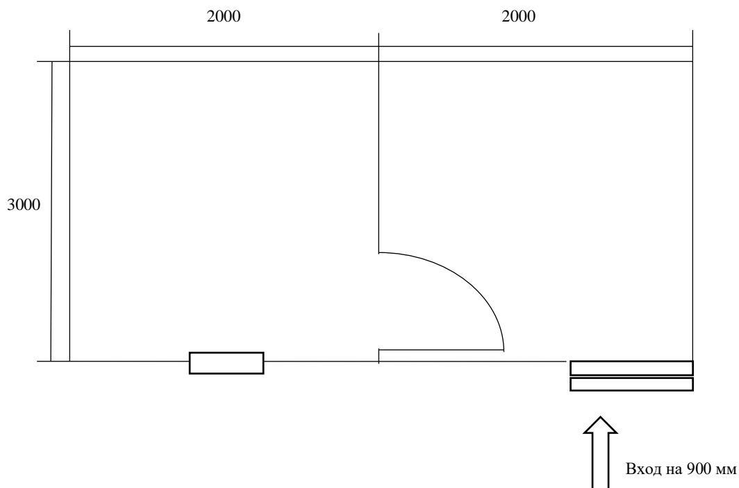
План-схема хозяйственного блока, совмещённого с беседкой р-р 3000х4000 мм
