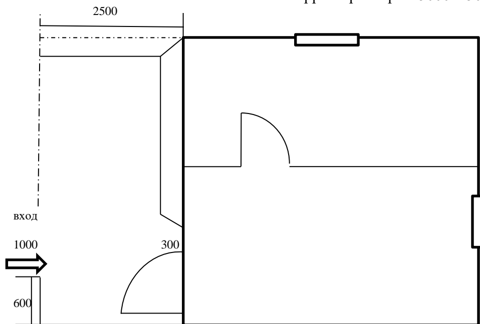
План-схема террасы размером 5000x2500 мм
