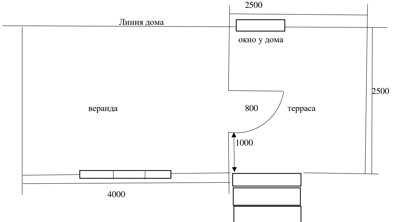
Спецификация на веранду р-р 4000х2500 мм с террасой р-р 2500х2500 мм, арт. 202
