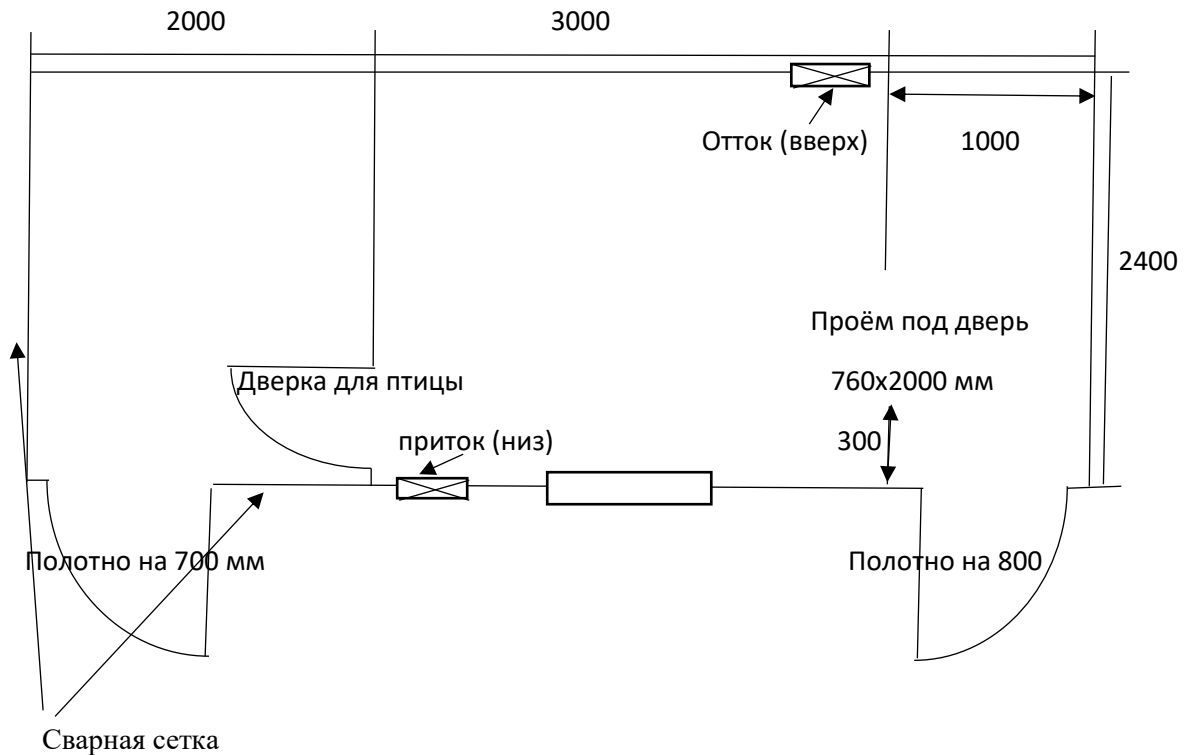
Курятник р-р 6х2,4 «Пташка» План-схема курятника р-р 6000х2400 мм
