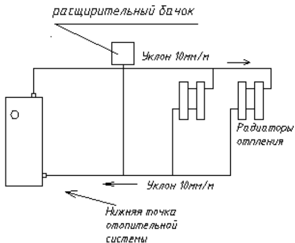
Рис.1 Схема монтажа открытой системы отопления.
