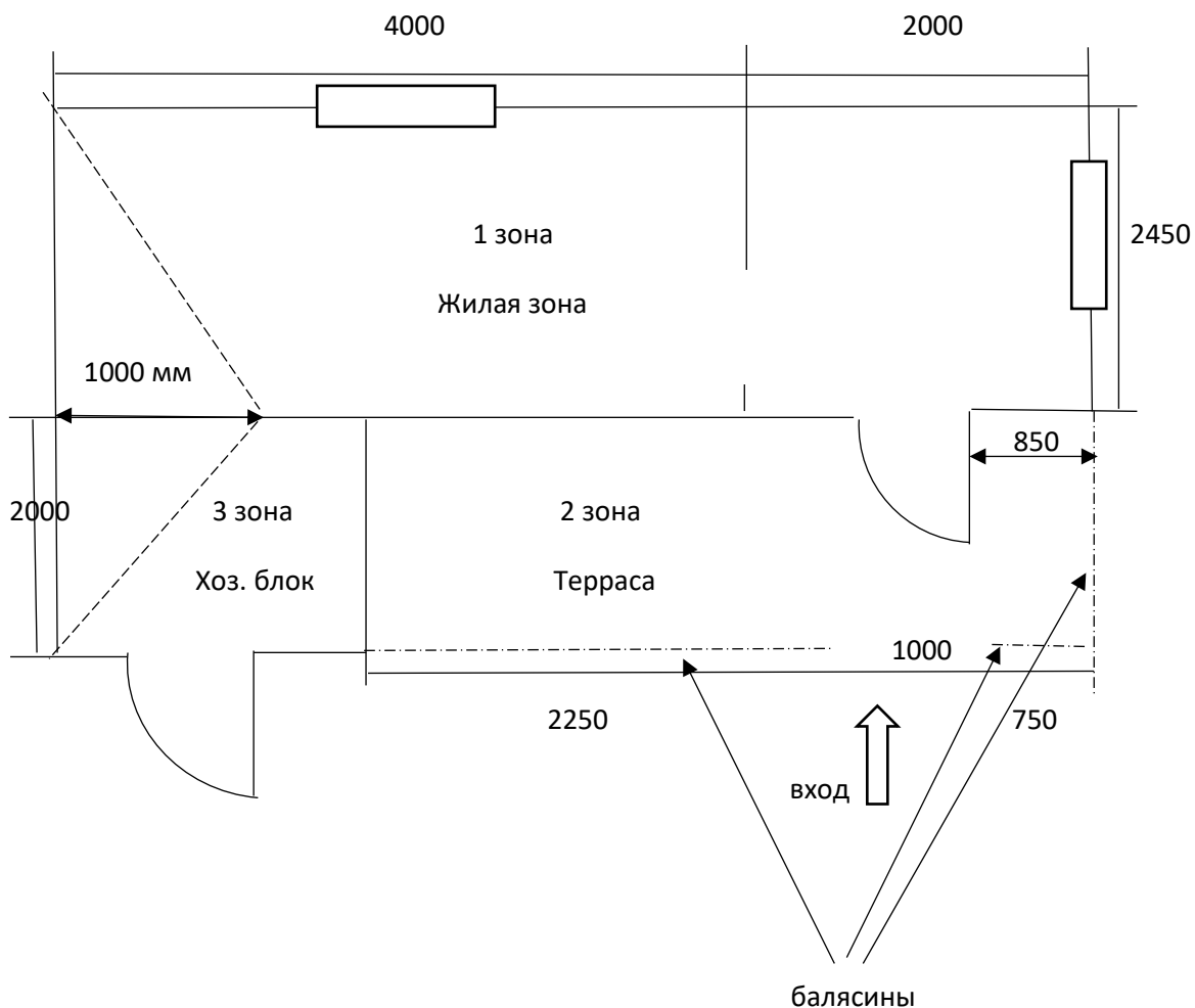
Спецификация на садовый домик р-р 6000x4900 мм, арт. 026
