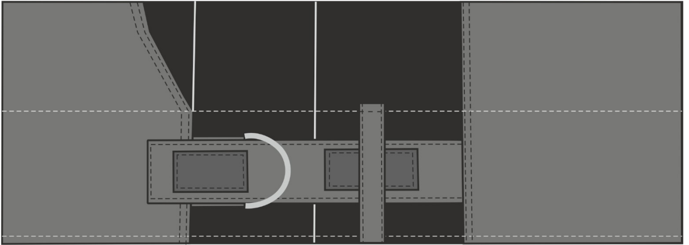
Рис.3.Эскиз Формула (тк.Смесовая,240) брюки, серый/красный/черный. Фрагмент бокового шва.
