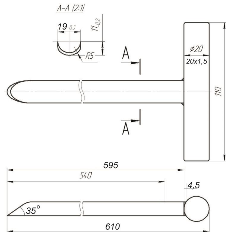
Рис.1 Щуп ПП СМ-540.
